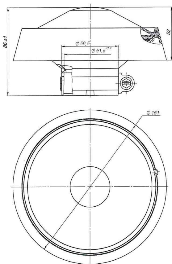
Моноциклон ИЖКС.061331.003
